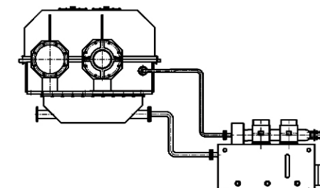
JDX 系列减速机油站连接示意图
