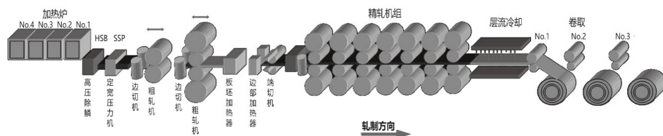
热轧板轧制工艺与减速机布置图
