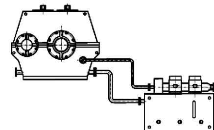
MBY 系列减速机油站连接示意图
